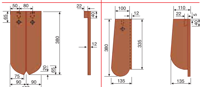
1/2 bobrovec, deljiv 18/38 okrogli rez
