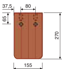
Slemenski bobrovec 15,5/27 Berlinski bobrovec
