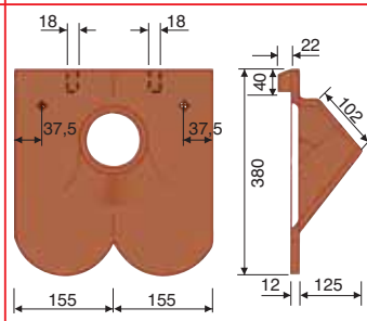
Bobrovec prehodni strešnik 31/38 Berlinski bobrovec
