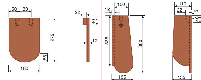
Slemenski bobrovec 18/27,5 okrogli rez
